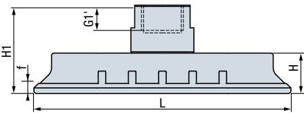
F38G/F38GA Fijación hembra G3/8"
