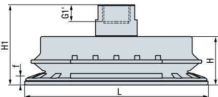
F38G/F38GA Fijación hembra G3/8"
