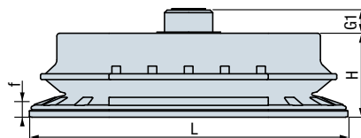
M38G Fijación macho G3/8"
